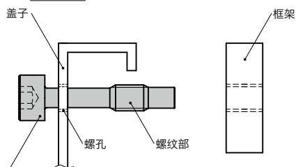
SSC-IG 内六角防脱落螺丝 (防偏斜拧紧)
