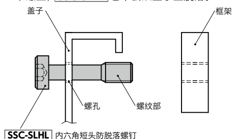
SSC-SLHL 内六角短头防脱落螺钉
