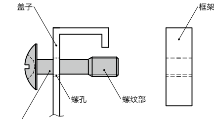
SSCML 十字槽防脱落伞头小螺钉
