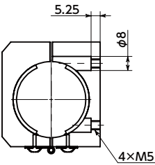
截面图 A-A
