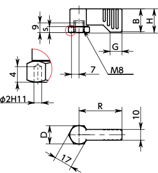
LSLK-B 内螺纹型
