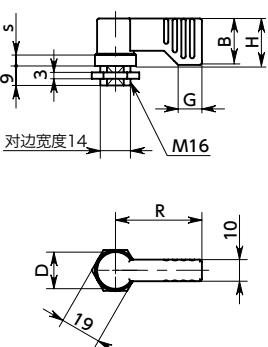
LSLK-C 外螺纹型
