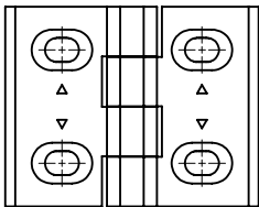
HND-B 水平方向调整型
