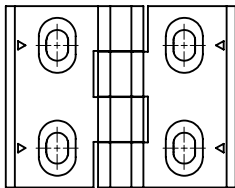
HND-H 垂直方向调整型
