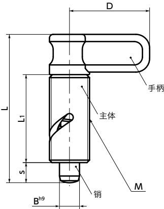
PDV-AK
