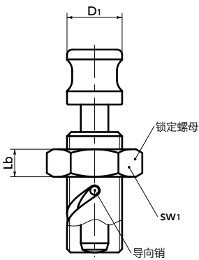
PDV-AK
