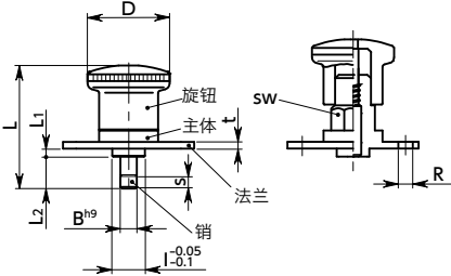
PFHY 主体、法兰：锌压铸件制/旋钮：塑料制
