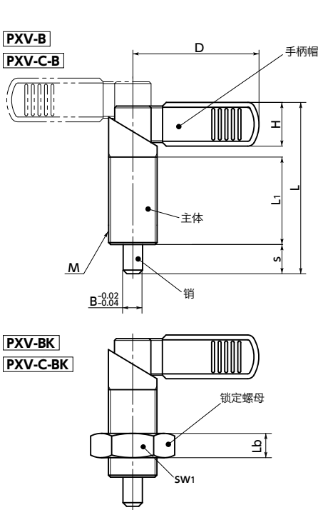
PXV-B 细牙螺纹、无锁定螺母 PXV-C-B 粗牙螺纹、无锁定螺母
