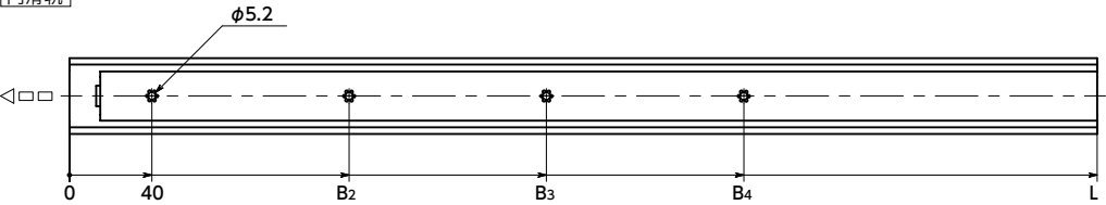
内滑轨
