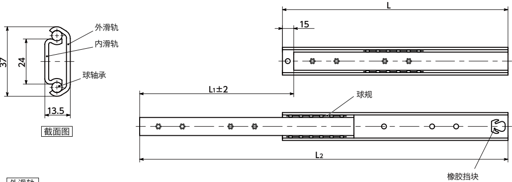
外滑轨
