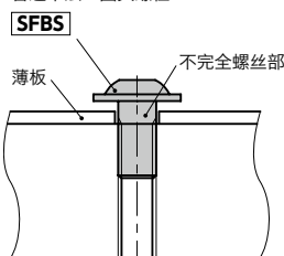
普通带法兰圆头螺栓
