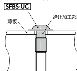
薄板固定用带法兰圆头螺栓
