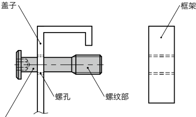
SSCHS-SD 内六角极短头小头防脱落螺钉
