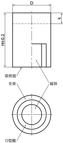
JST-AN-TZB 铝镍钴，外径公差D ±0.1
