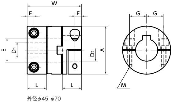
外径φ45-φ70
