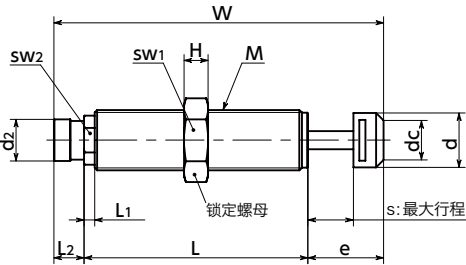
PAE-□H□S
