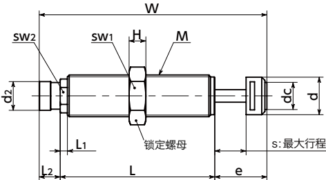
PAE-□H□K
