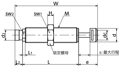
PAE-□H□K
