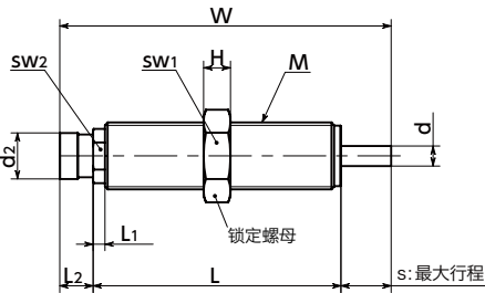
PAE-□H□S
