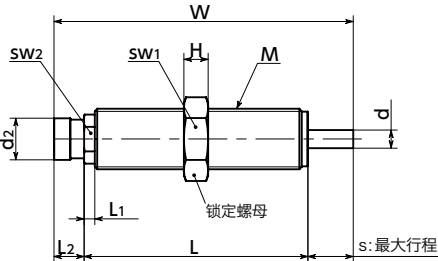
PAE-□H□S
