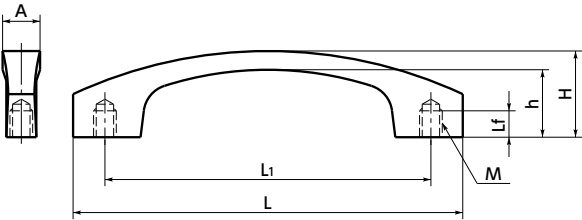
TC 内螺纹
