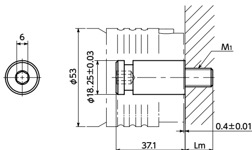
外螺纹型
