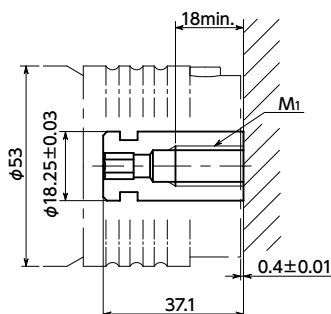
内螺纹型
