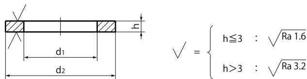
小型－零件等级A的形状
