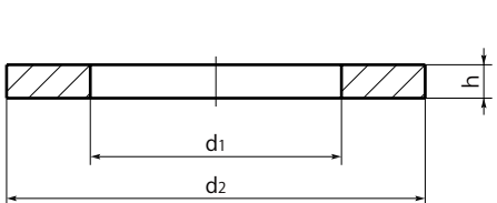
普通型－零件等级C的形状
