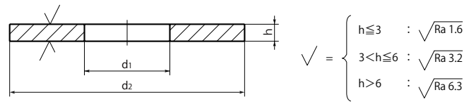
大型－零件等级A的形状
