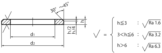
普通型倒角－零件等级A的形状
